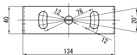
ヨーク取付け穴寸法
