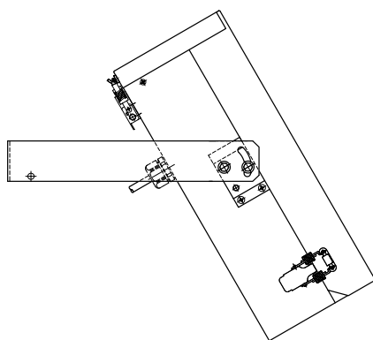
ヨーク取付部
